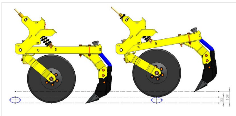
Sistema de deslocamento do facão em obstáculos
