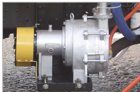
Bomba vácuo e pressão de anel líquido de 8 m 3 /min ou 12 m 3 /min vazão de ar
