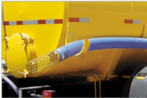
Mangueira de carga
