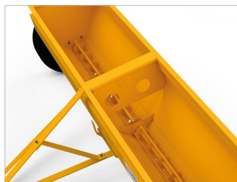
Sistema de distribuição com rotor agitador.
